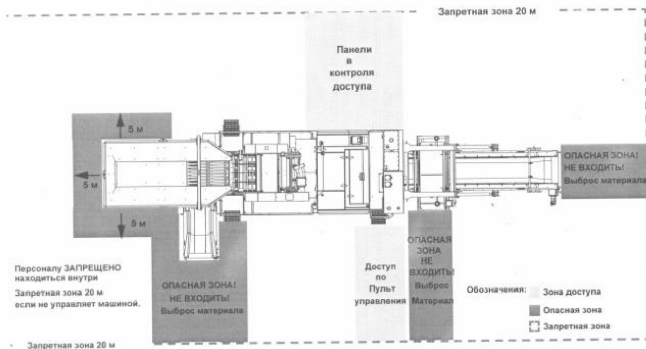
Рисунок 5 Опасные зоны при работе щековой дробилки
