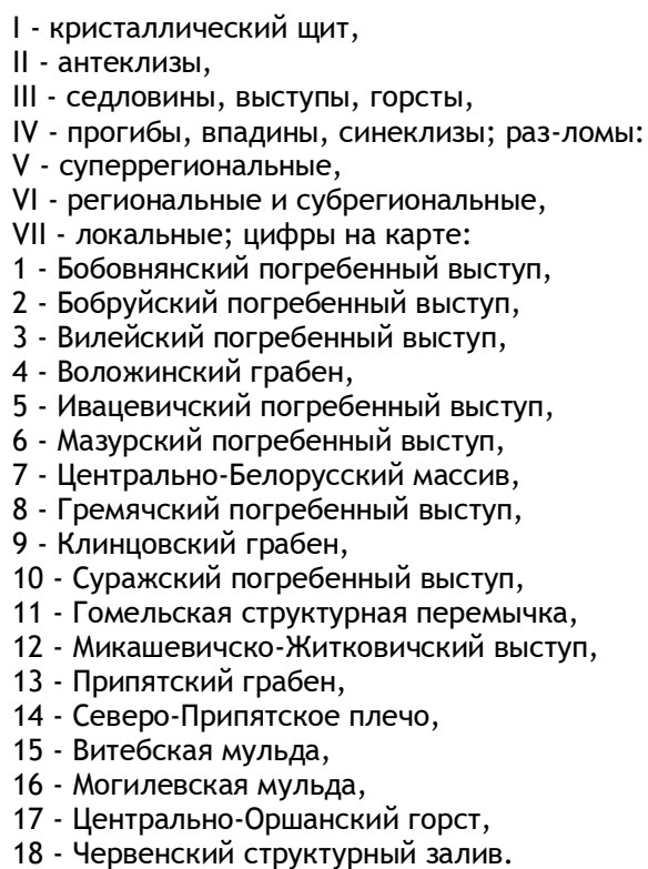
Рисунок 3 Карта тектонического районирования территории Беларуси
